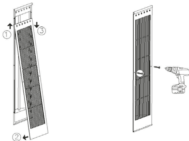
Abbildung 37: Montage der Abdeckgitter
