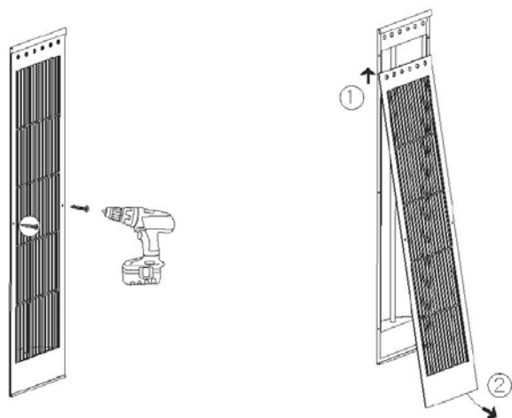
Abbildung 36: Demontage der Abdeckgitter
